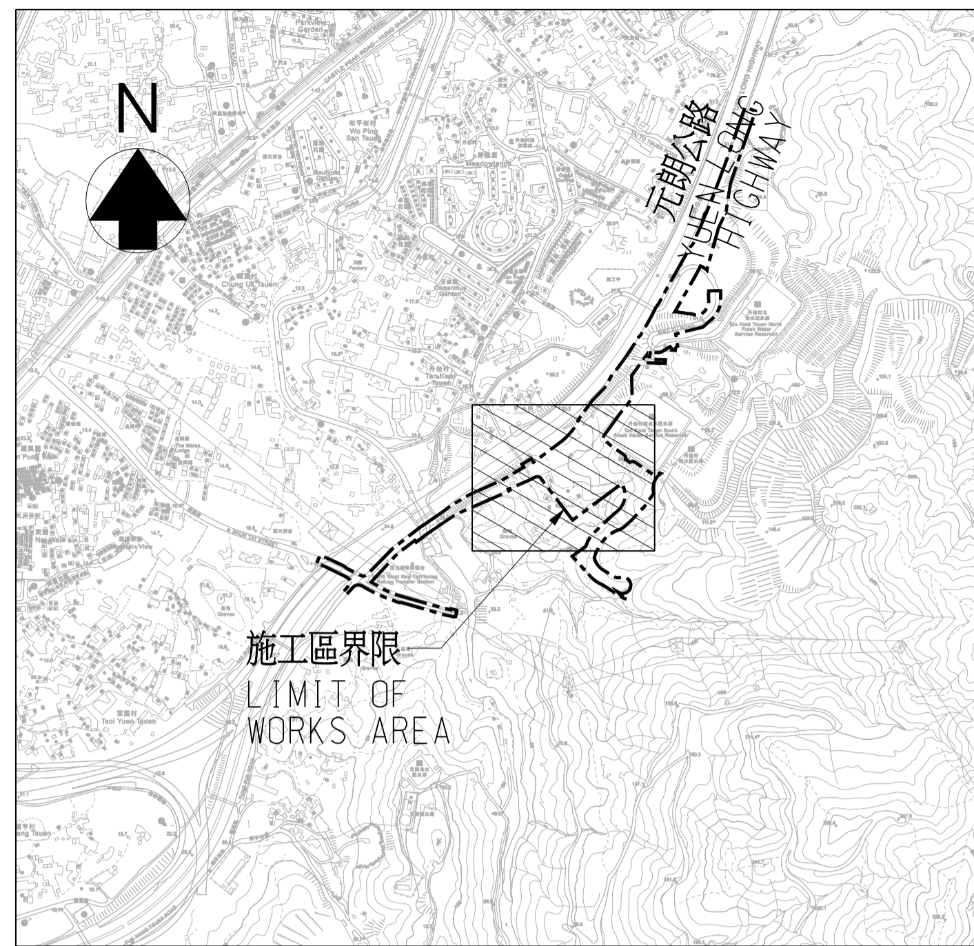
KEY PLAN 索引圖 比例 SCALE A3 1 : 20000
