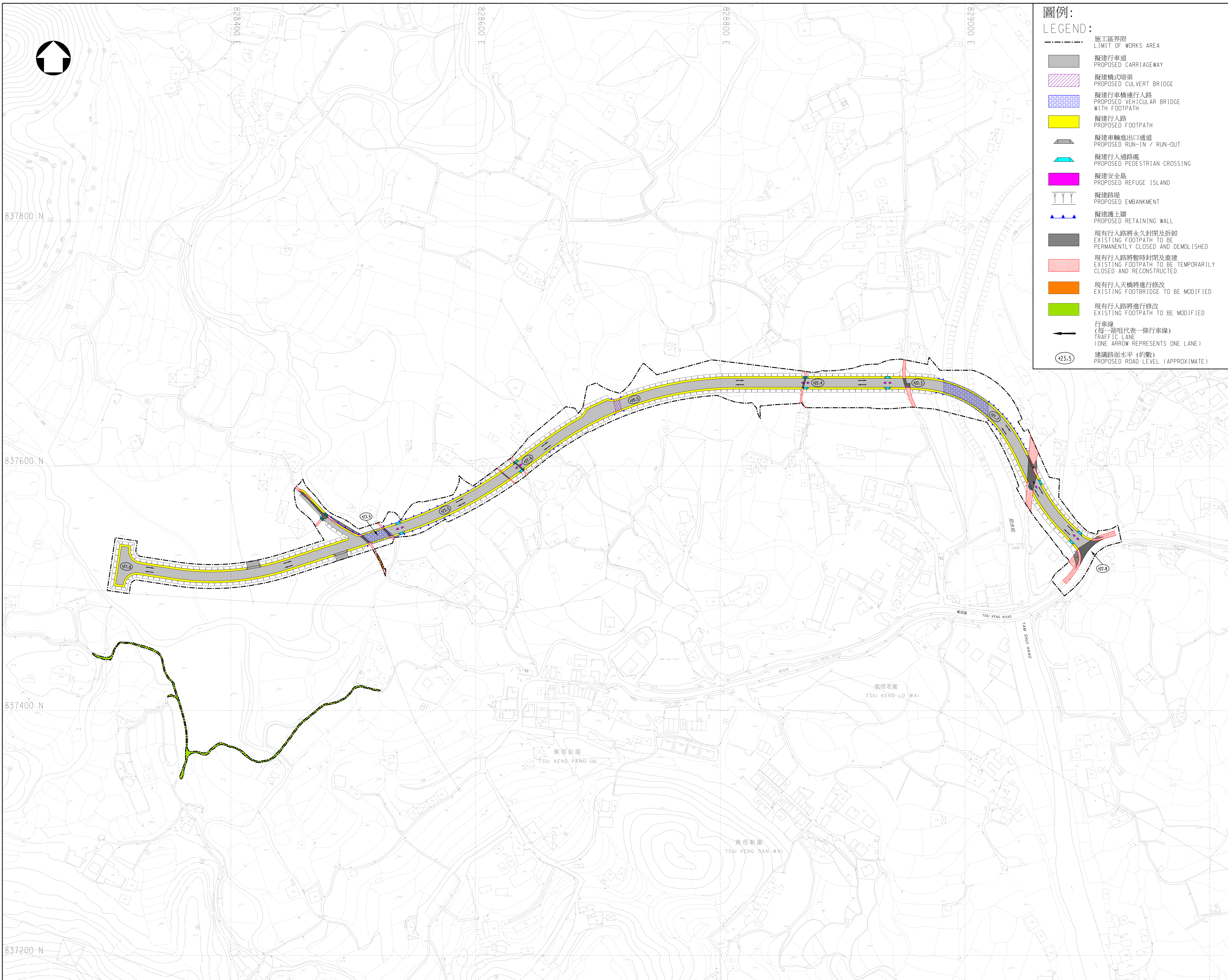
位置圖 LOCATION PLAN 比例 1:10000 SCALE 1:10000
