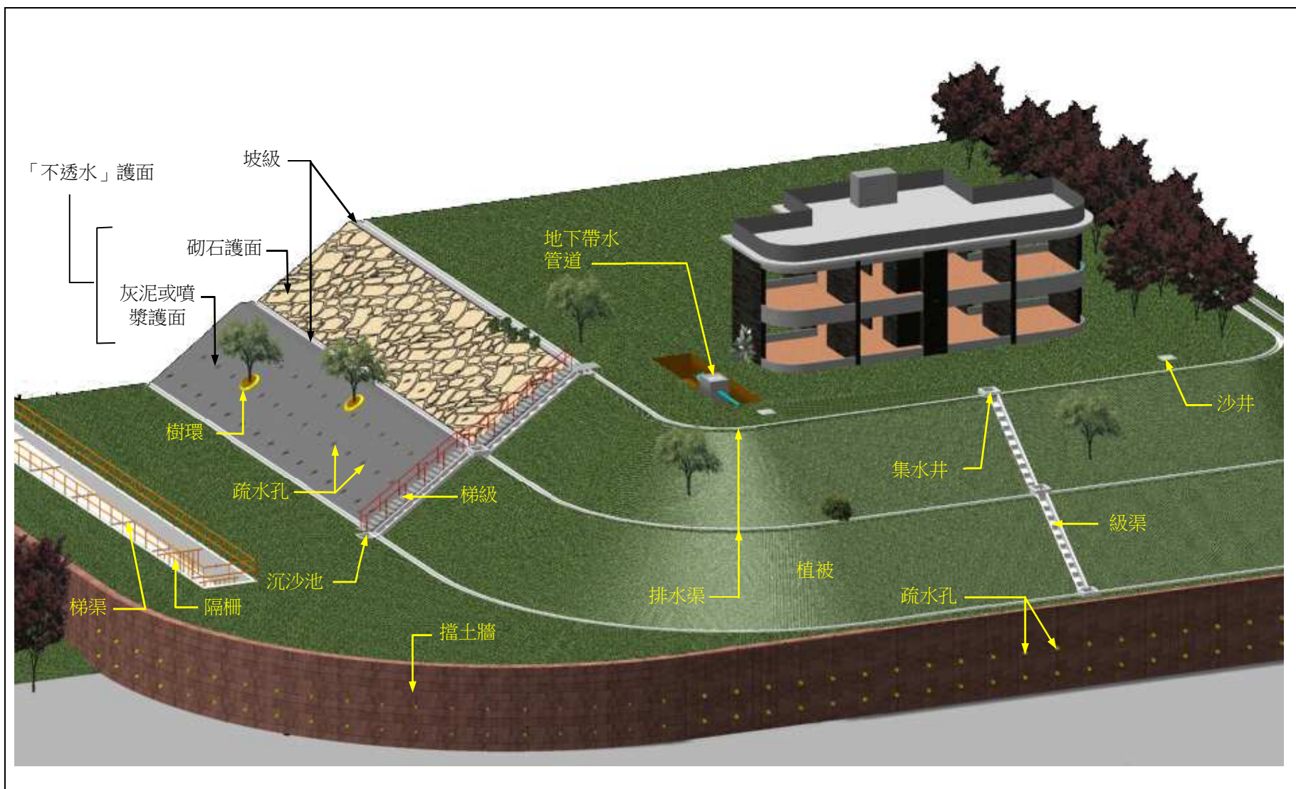
圖3.1 斜坡及擋土牆上一般需維修的人造設施
