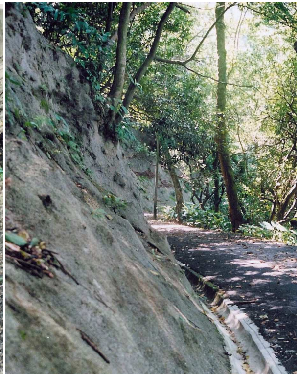
(2) 噴漿混凝土護面
