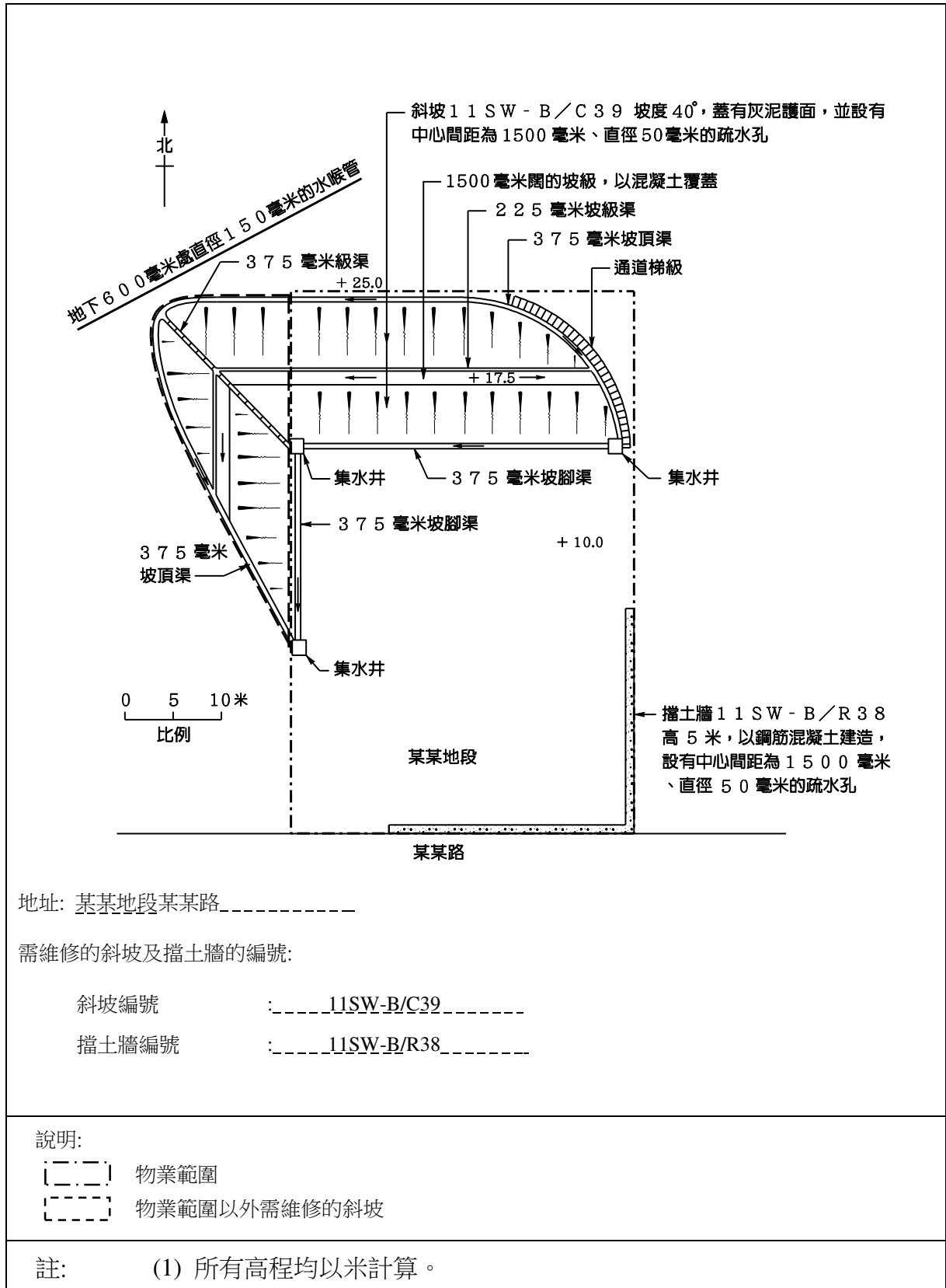
圖 2.1 需維修的斜坡及擋土牆的典型平面圖
