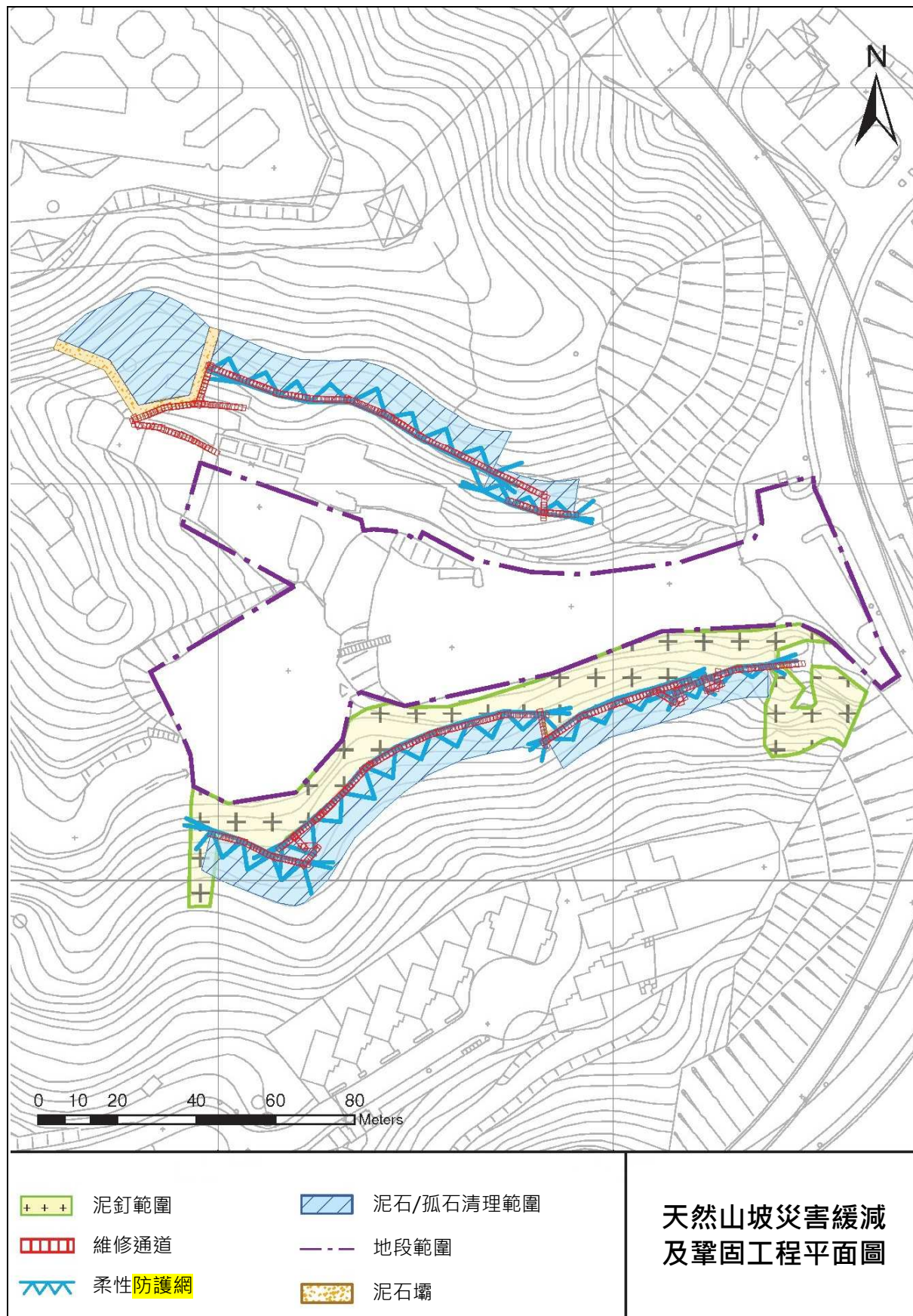
圖 1.2 於土地註冊處登記的典型天然山坡災害緩減及鞏固工程平面圖
