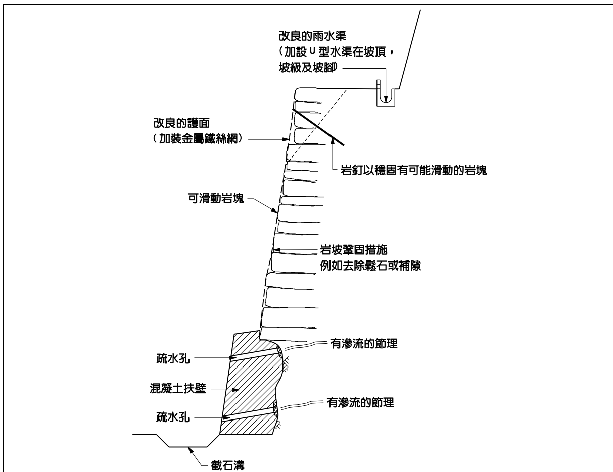
圖 5.2 典型的岩石坡預防性維修工程
