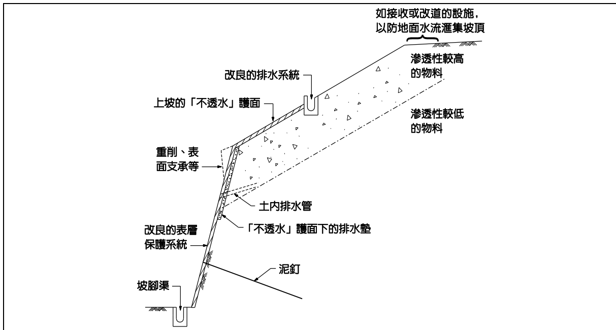
圖 5.1 典型的削土坡預防性維修工程
