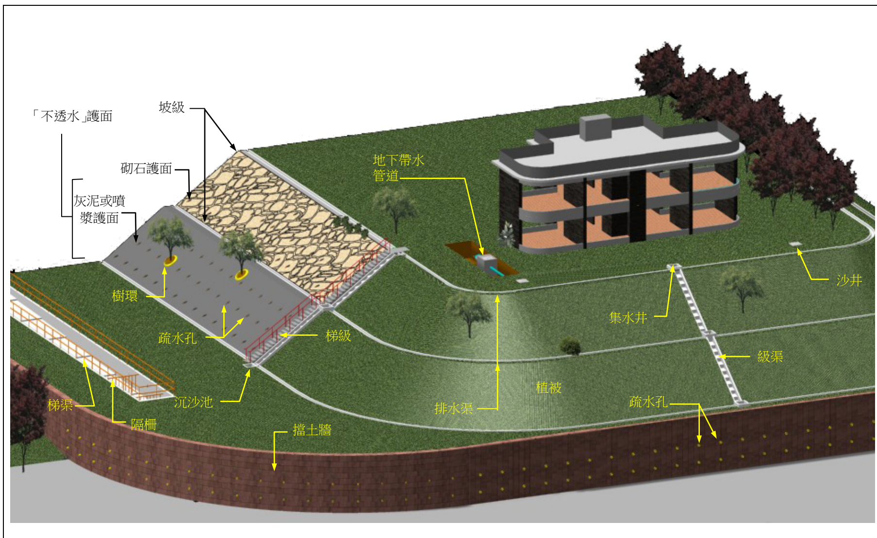
圖3.1 斜坡及擋土牆上一般需要維修的設施
