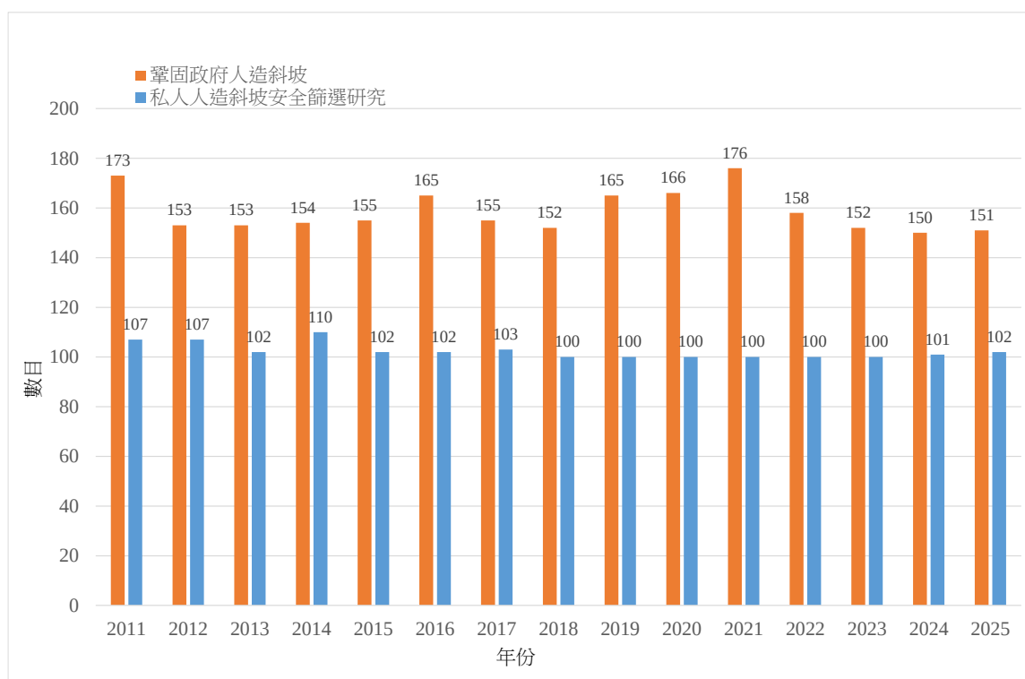
圖 1 - 2011 至 2025 年「防治計劃」下每年完成的政府人造斜坡鞏固工程及私人人造斜坡安全篩選研究的數目
