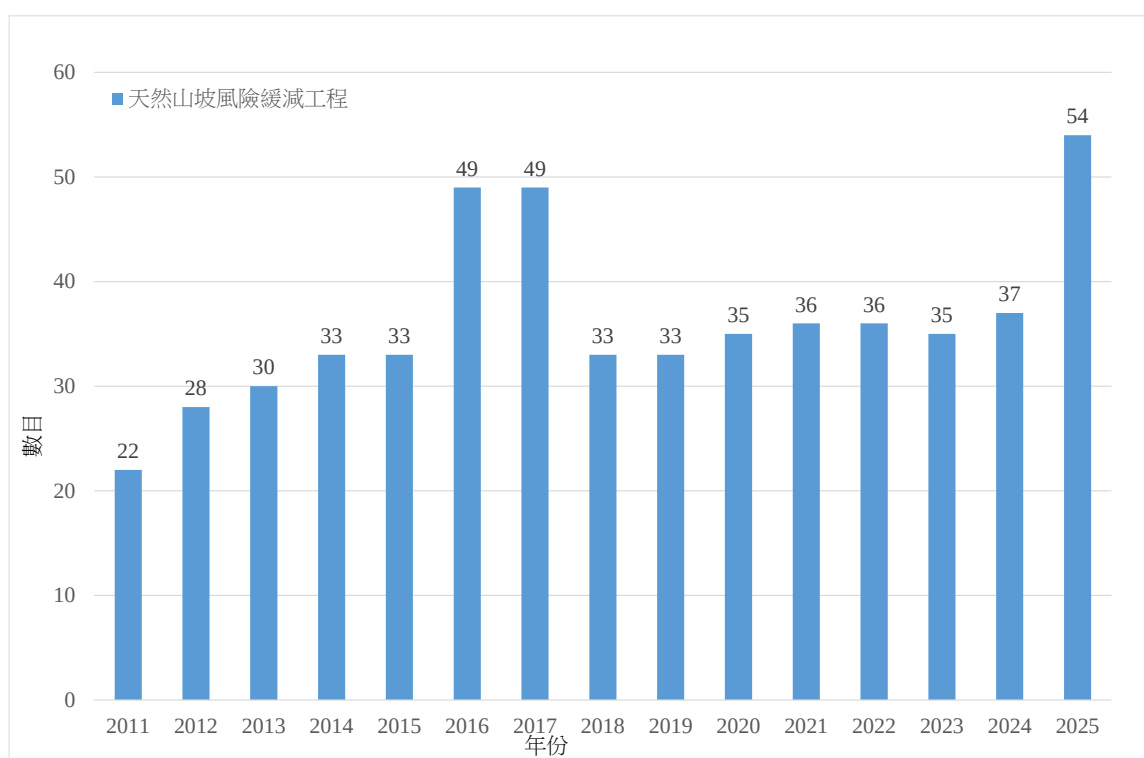
圖 2 - 2011 至 2025 年「防治計劃」下每年完成的天然山坡風險緩減工程數目
