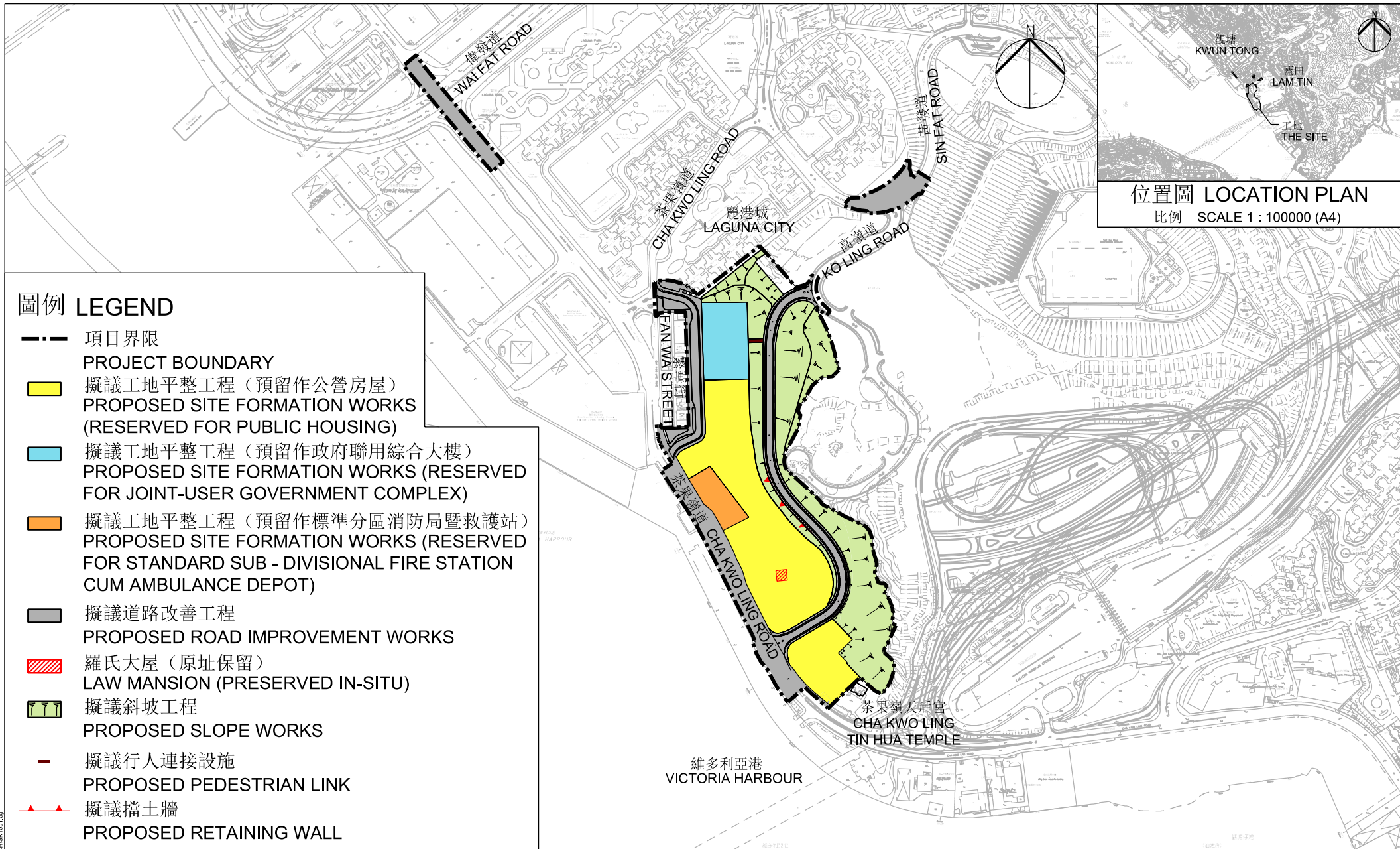
工地平面圖 SITE PLAN 比例 SCALE 1:6000 (A4)
