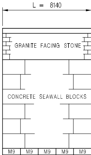
ELEVATION
