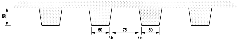
DEEP RIB PATTERN SCALE 1 : 5
