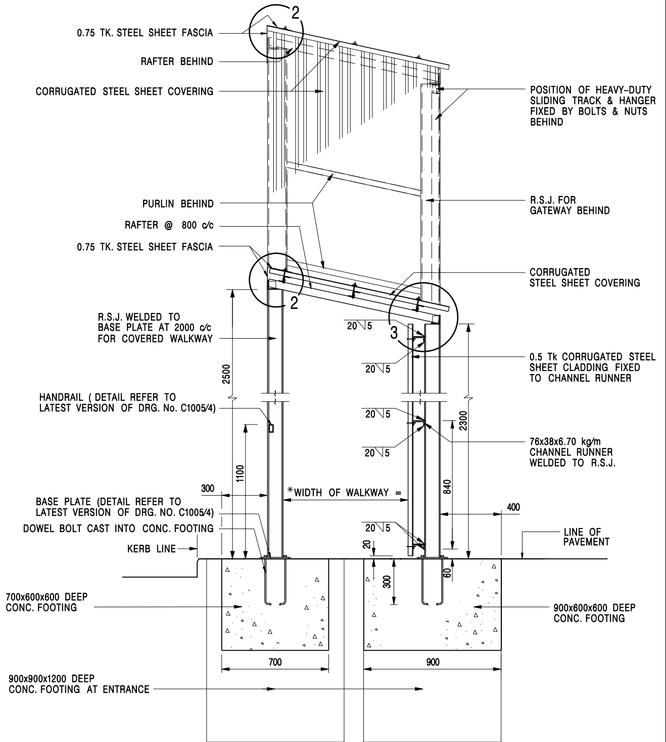
SECTION A-A
