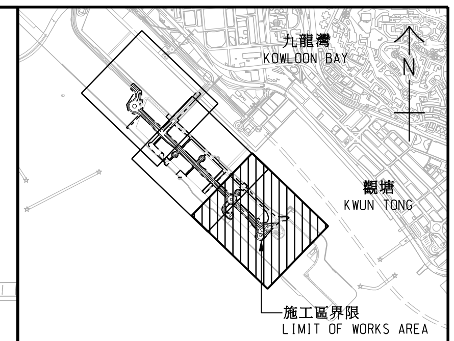
位置圖 LOCATION PLAN 比例 SCALE A1 1 : 25000
